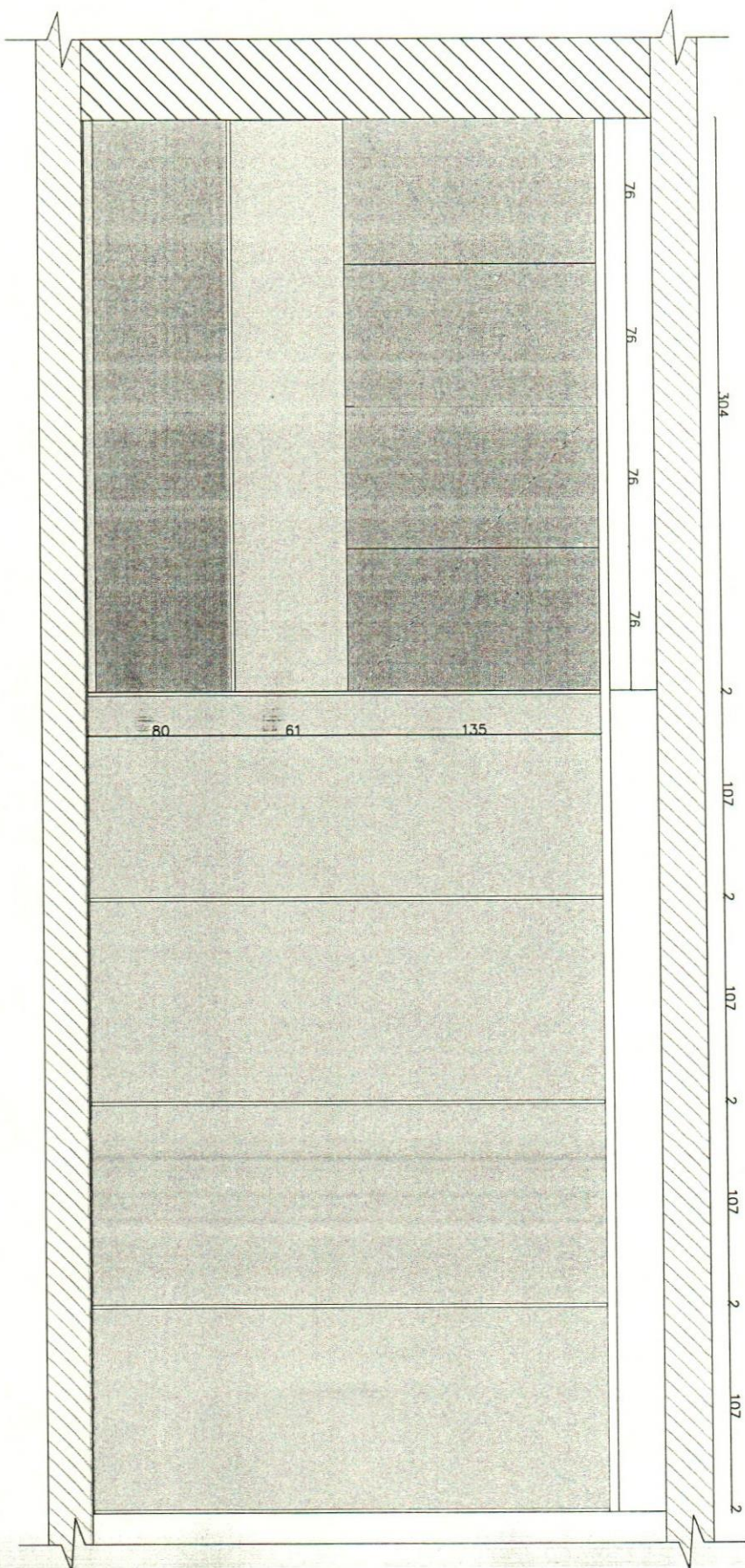
المهندس طوني صليبا SECTION B SIXTH FLOOR WOOD WALL UNIT
