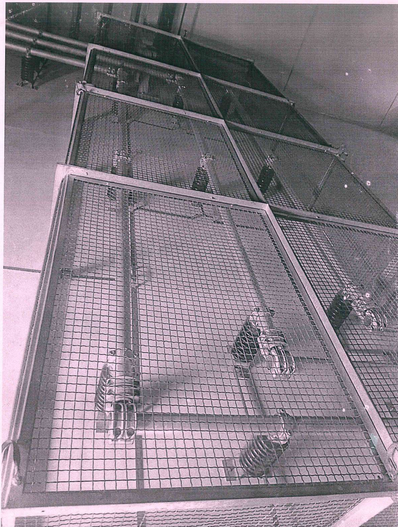
(4000A) Jeux de barres 24 KV - 85 -
